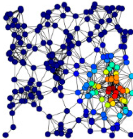
Mapa de calor utilizando a métrica de PageRank
