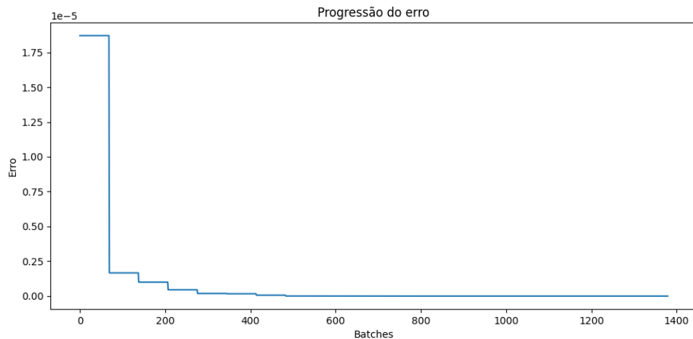
Perda ( loss ) do algoritmo de rede neural ao longo do treinamento
