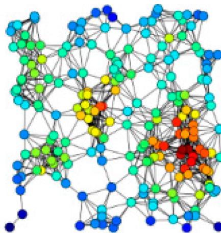
Exemplo de nós com maior grau de entrada (mapa de calor)
